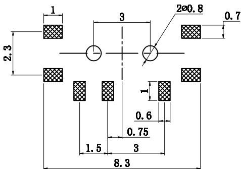
安装参考图
