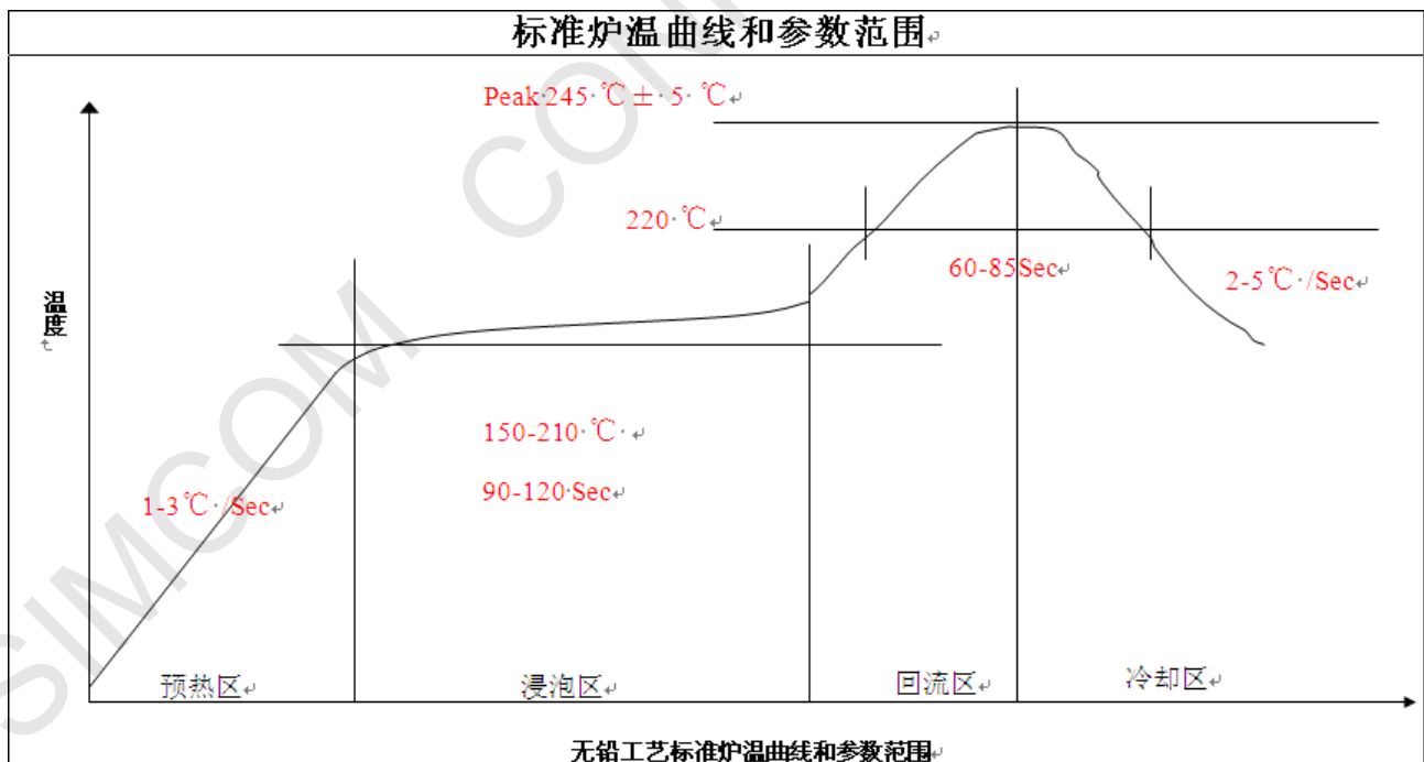
图 53: 模块推荐焊接炉温曲线图（无铅工艺）
