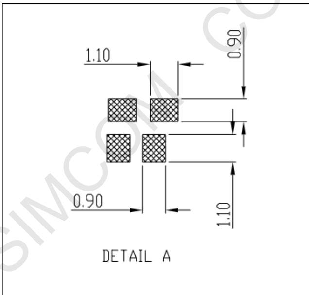
图 4：推荐 PCB 封装尺寸（单位：毫米）
