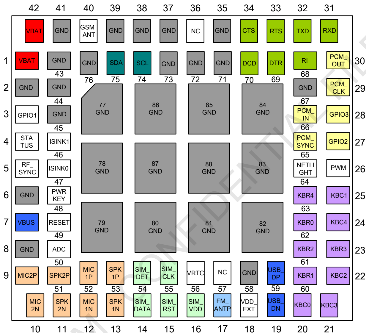
图 2: 模块引脚图(TOP 面透视图)
