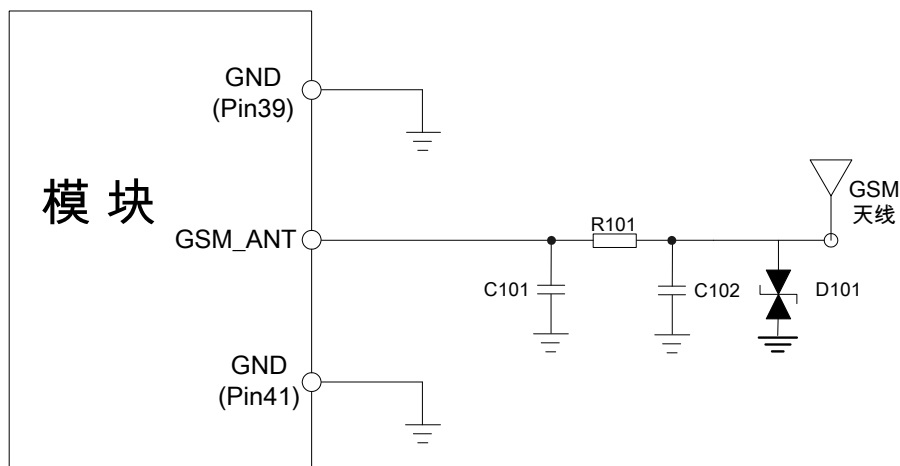
图 47：GSM 天线接口简化连接电路
