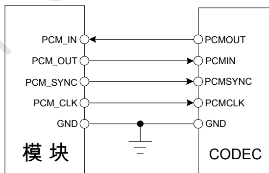
图 36: PCM 连接图
