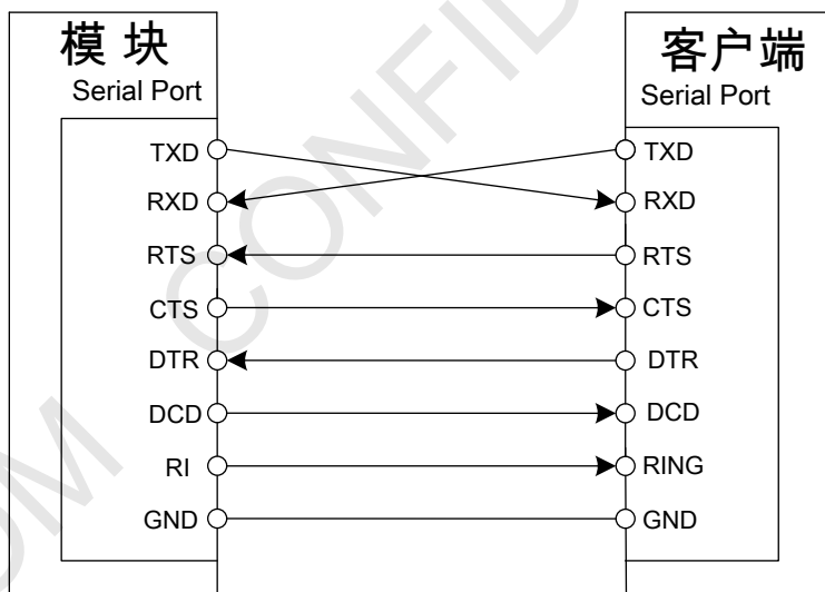
图 20：串口连接图
