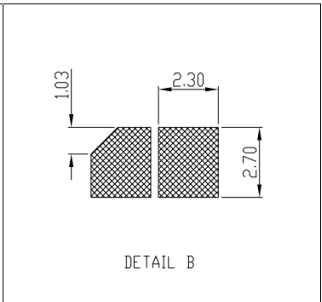
图 4：推荐 PCB 封装尺寸（单位：毫米）
